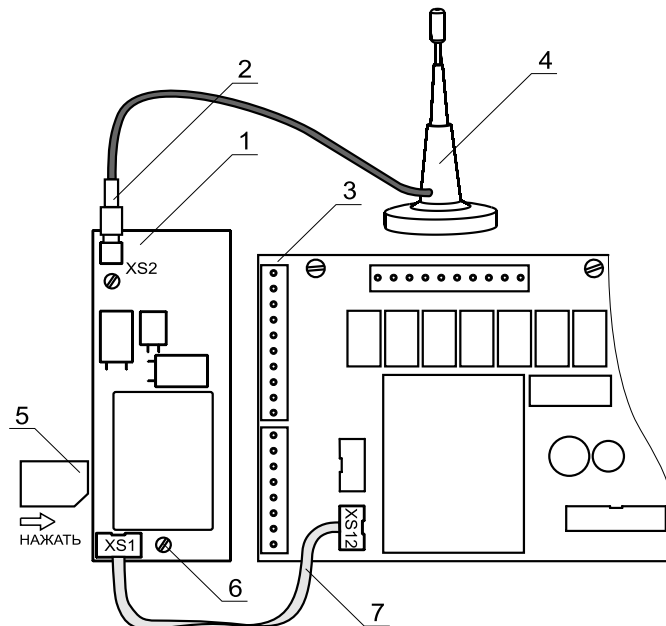
Рис.1 Конструкция и подключение модуля GSM
